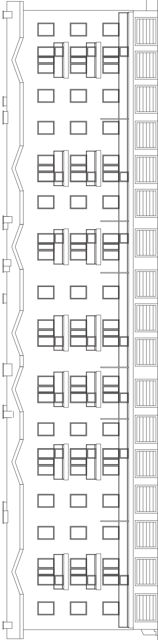
Elewacja wschodnia
